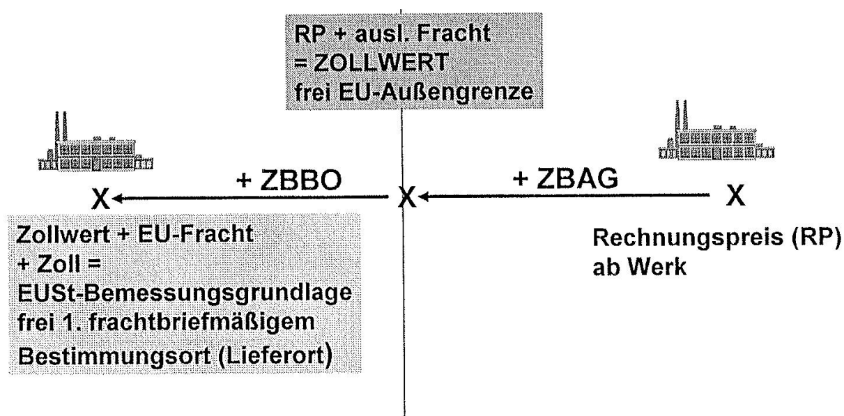
Abbildung 3: Berechnung EXW
