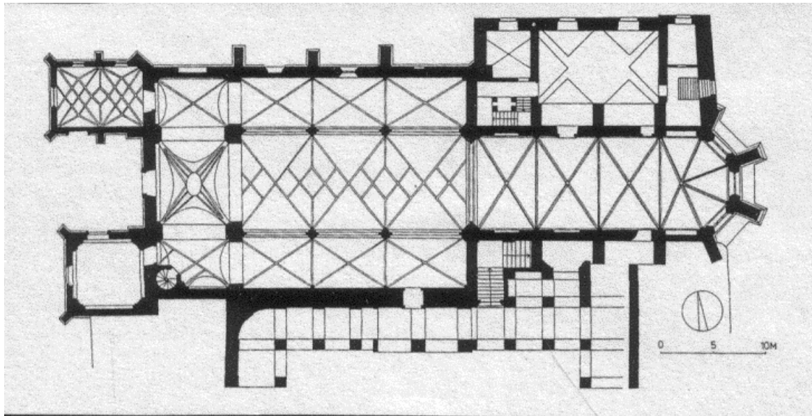
Abb. 23: Wiener Neustadt, Kirche des ehemaligen Zisterzienserstiftes Neukloster, Grundriss
