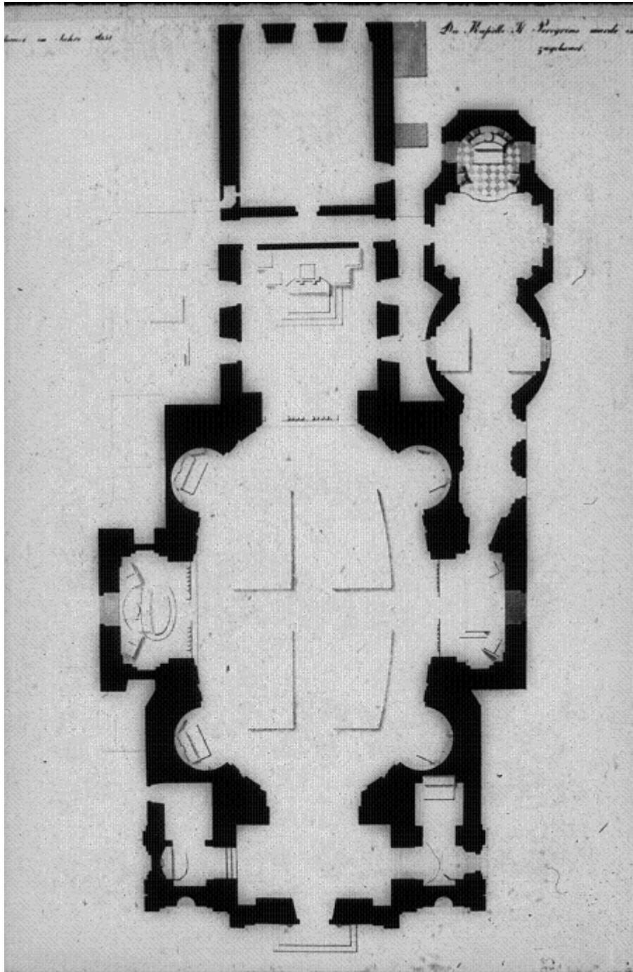
Abb. 58: Wien, Servitenkirche, Grundriss
