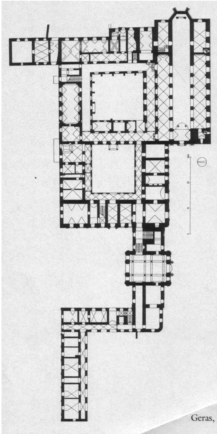
Abb. 4: Geras, Prämonstratenserstift Geras, Grundriss
