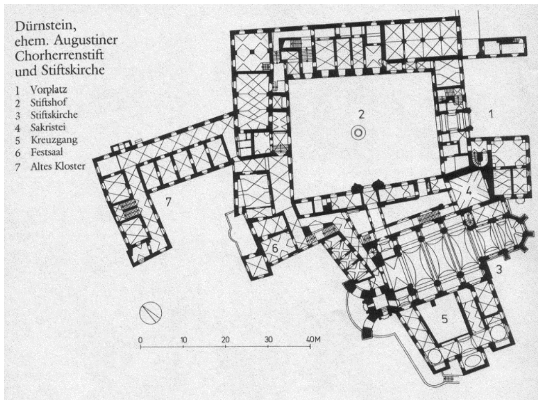
Abb. 30: Dürnstein, Ehemaliges Augustiner-Chorherrenstift Dürnstein, Grundriss
