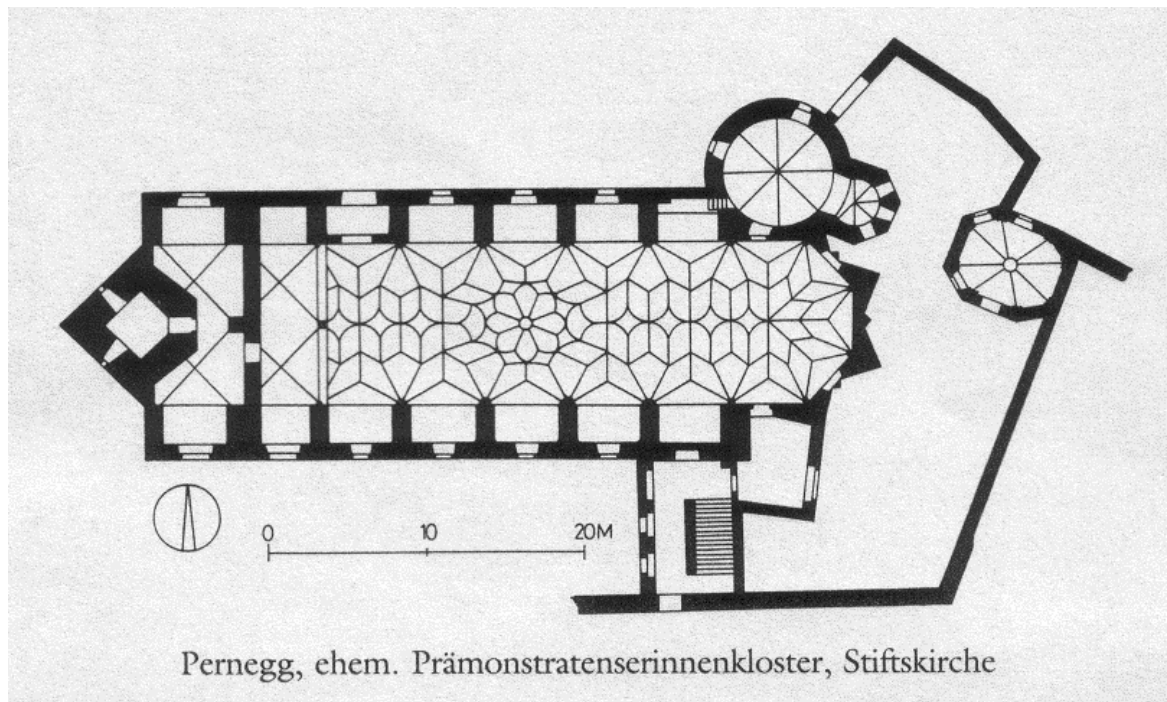
Abb. 34: Pernegg, Kirche des ehemaligen Prämonstratenserstiftes Pernegg, Grundriss
