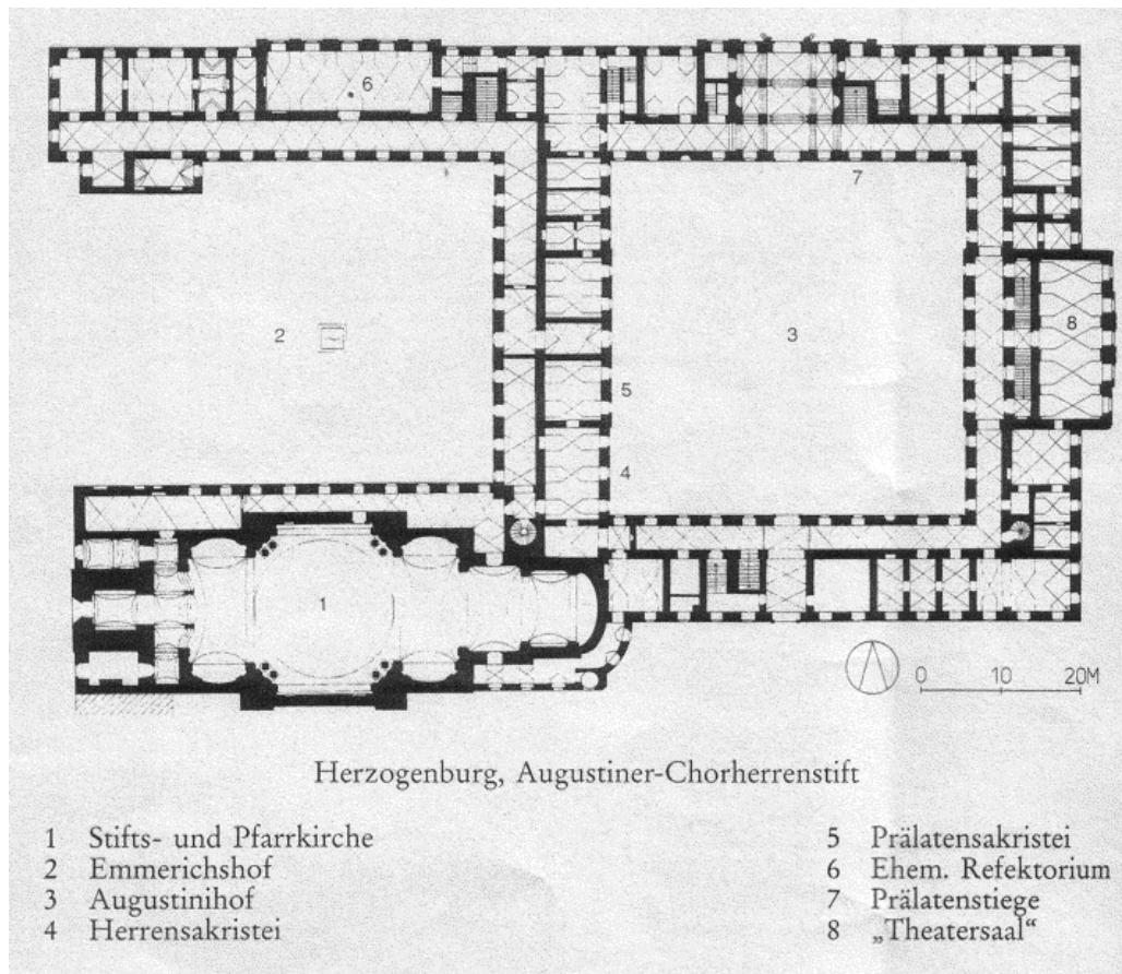
Abb. 12: Herzogenburg, Augustiner-Chorherrenstift Herzogenburg, Grundriss
