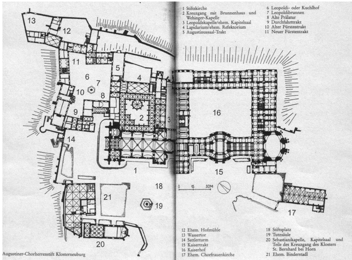
Abb. 14: Klosterneuburg, Augustiner-Chorherrenstift Klosterneuburg, Grundriss
