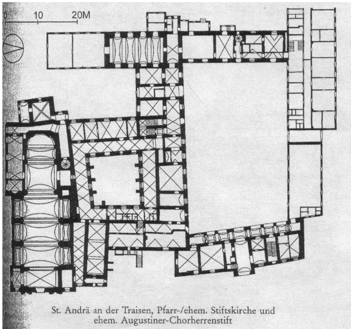
Abb. 36: St. Andrä a. d. Traisen, Ehemaliges Augustiner-Chorherrenstift St. Andrä a. d. Traisen, Grundriss
