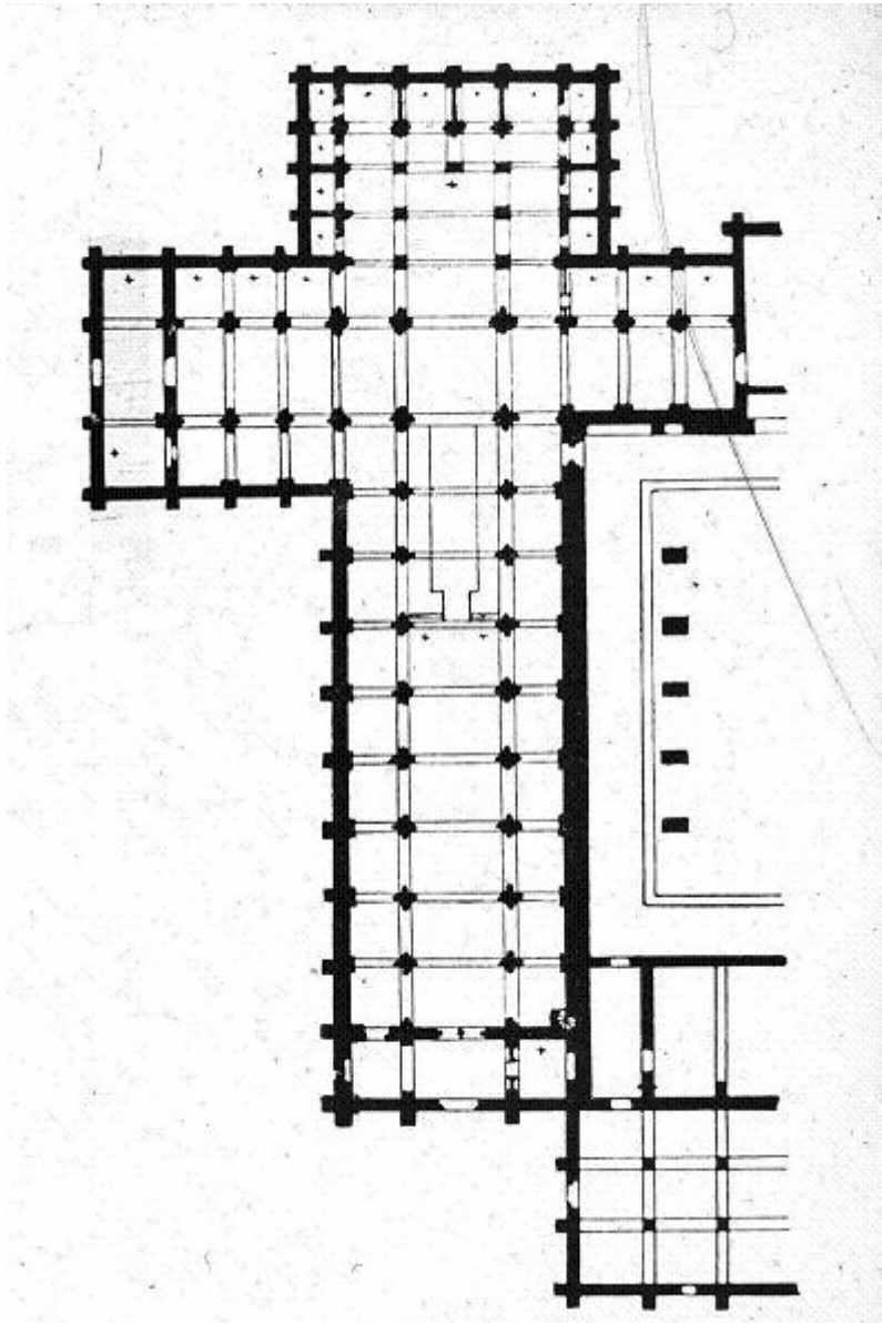
Abb. 56: Cîteaux, Abteikirche Cîteaux III (Weihe 1193), Grundriss
