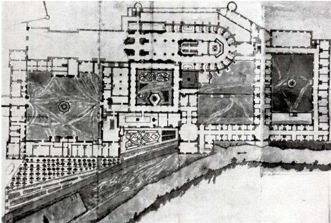
Abb. 27: Zwettl, Zisterzienserstift Zwettl, Grundriss, Bauplane Nr. VIII
