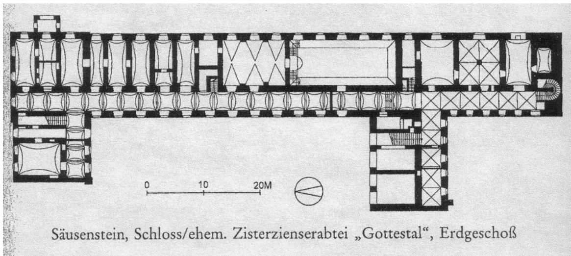
Abb. 40: Säusenstein, Ehemaliges Zisterzienserstift Säusenstein, Grundriss
