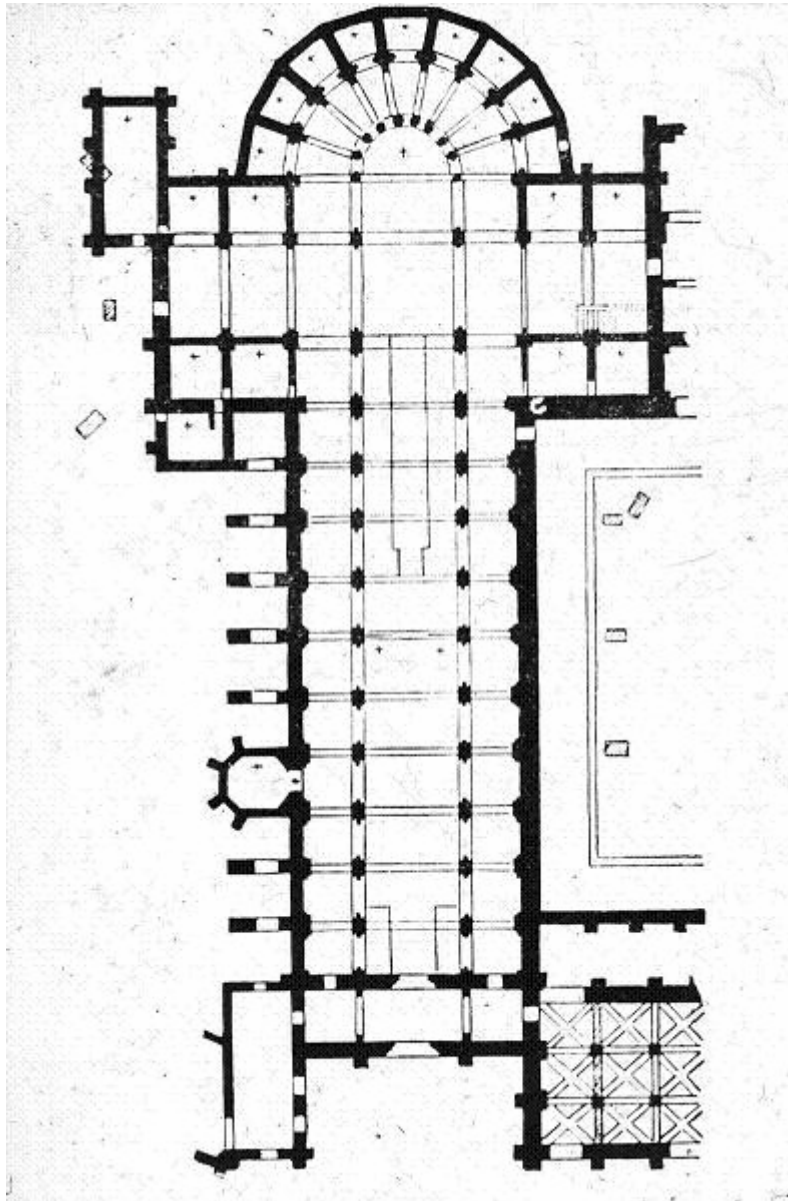
Abb. 57: Ville-sous-la-Ferté, Abteikirche Clairvaux III (1154 - 1174), Grundriss
