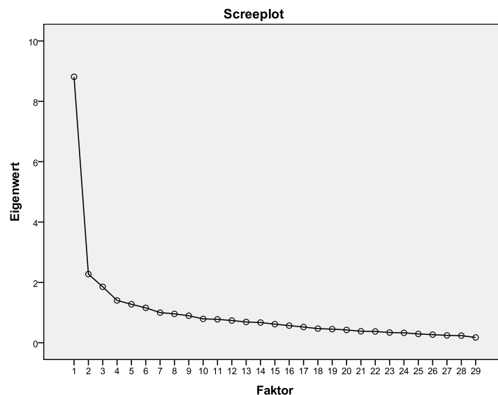
Abbildung 19: Screeplot; grafische Darstellung des Eigenwertverlaufs.
